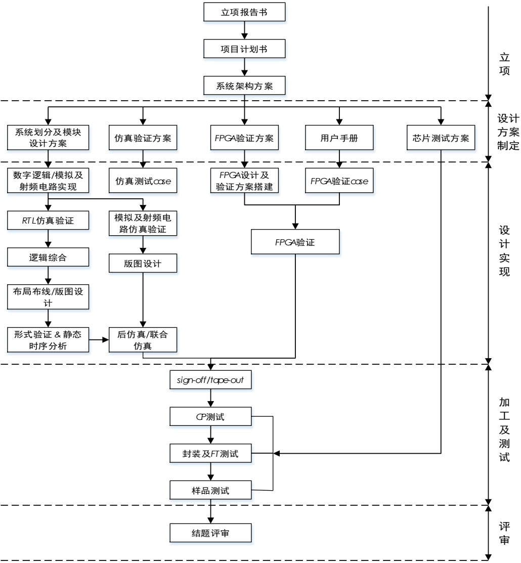
芯片设计开发项目执行流程图
